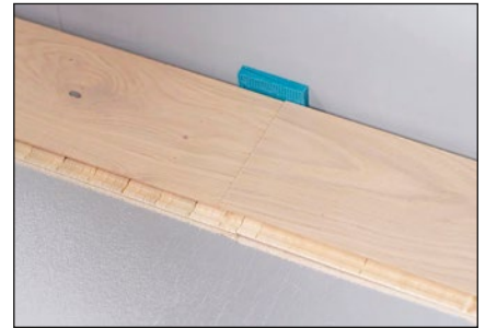
Mit Hilfe von den Kunststoff-Rastkeilen zu allen Wänden und festen Objekten im Raum einen Abstand von mindestens 10 bis 15 mm einhalten.
