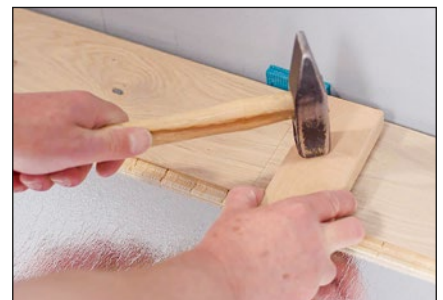
Fügen Sie die Kopffugen mit einem Hammer und Schlagschutz zusammen. Die Längs- und Kopffugen verriegeln dabei automatisch. Diese Verlegung im ganzen Raum fortsetzen.
