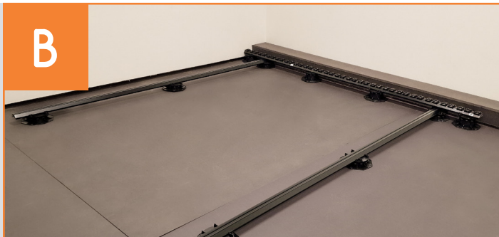
Erste Systemschiene positionieren
