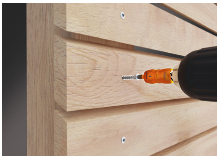
Fassadenverschraubung
