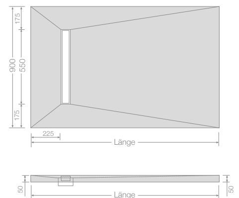
4-seitiges Gefälle
