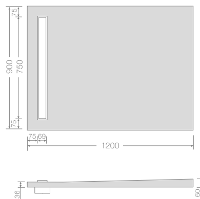
1-seitiges Gefälle
